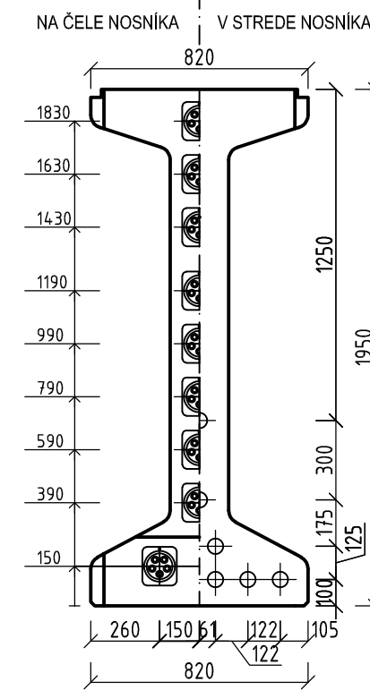
PRE DĹŽKU NOSNÍKA 42m (prosté pole)
