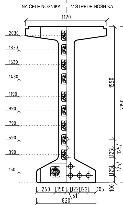
PRE DĹŽKU NOSNÍKA 42m (prosté pole)
