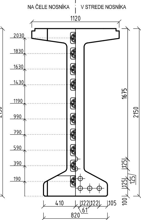
PRE DĹŽKU NOSNÍKA 42m (spojité polia)
